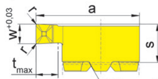
Klemmhalter Stirnseite Toolholder face
