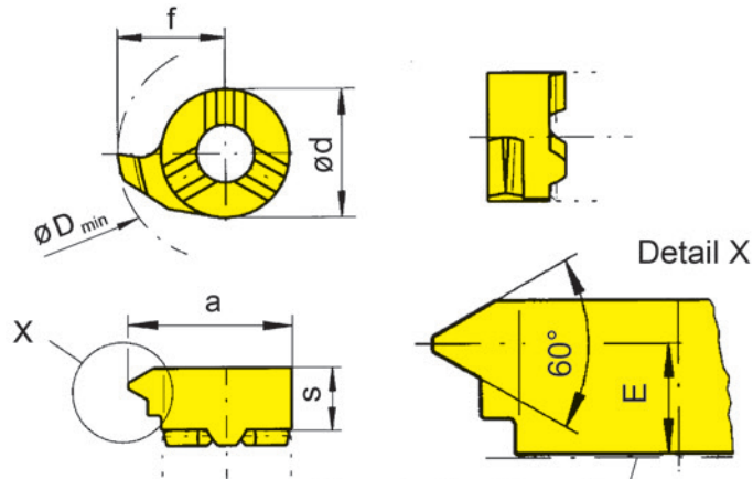
Klemmhalter Stirnseite
